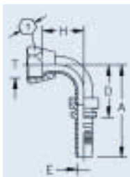
Skive Nipple
