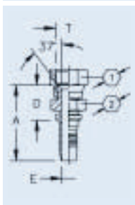
Skive Nipple
