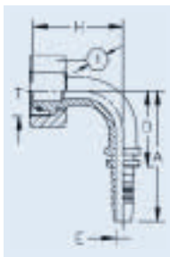
Skive Nipple
