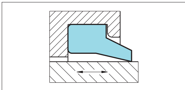
Bild 19 Abstreifer WRM
