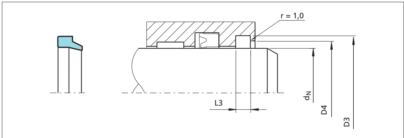
Bild 20 Einbauzeichnung
