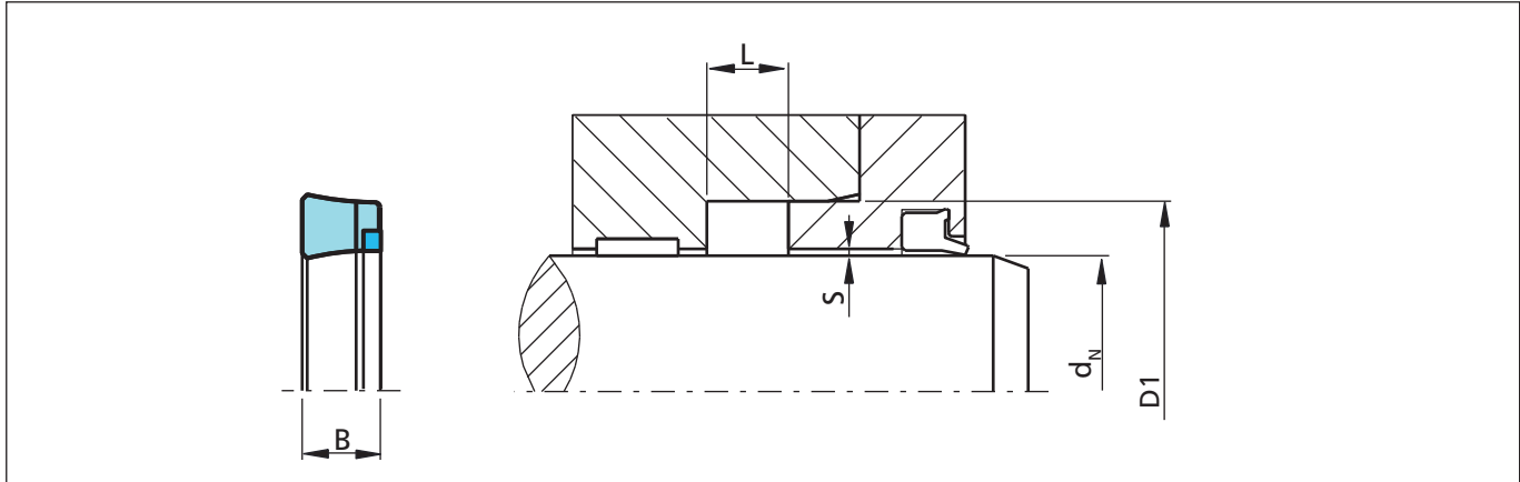
Bild 37 Einbauzeichnung
