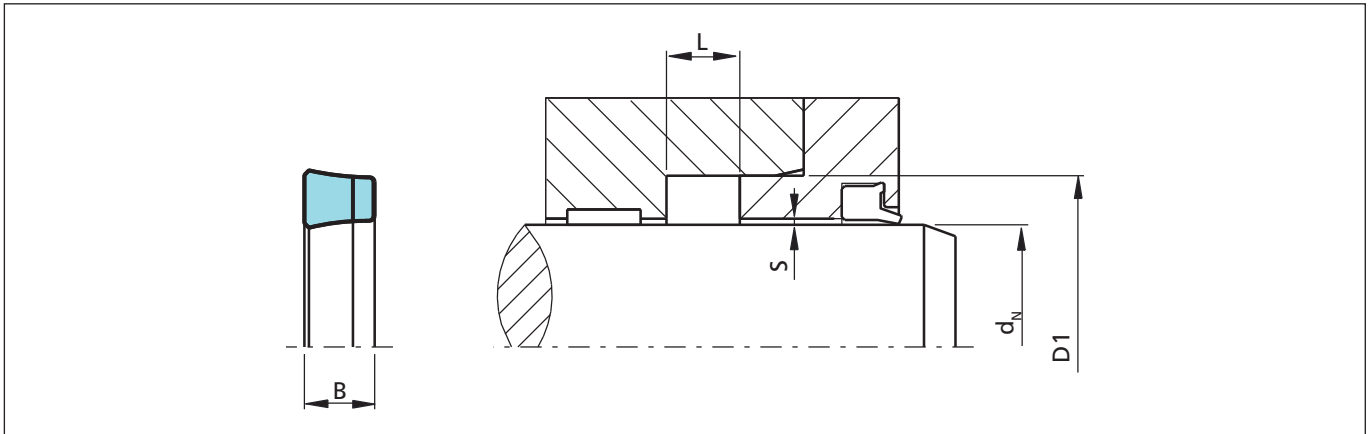
Bild 36 Einbauzeichnung
