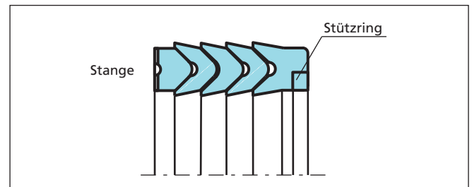
Bild 29 Veepac Ausführung mit Stützring
