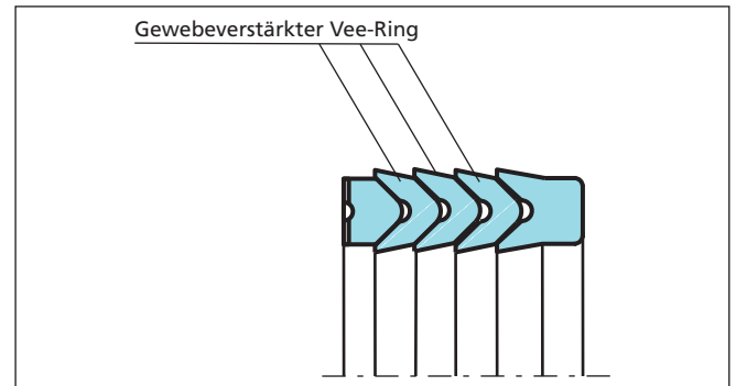
Bild 28 Veepac Ausführung mit 3 gewebeverstärkten Vee-Ringen
