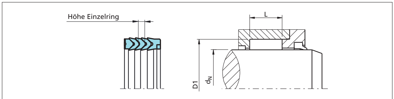
Bild 31 Einbauzeichnung
