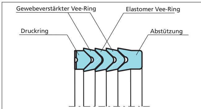
Bild 27 Veepac Standard Ausführung
