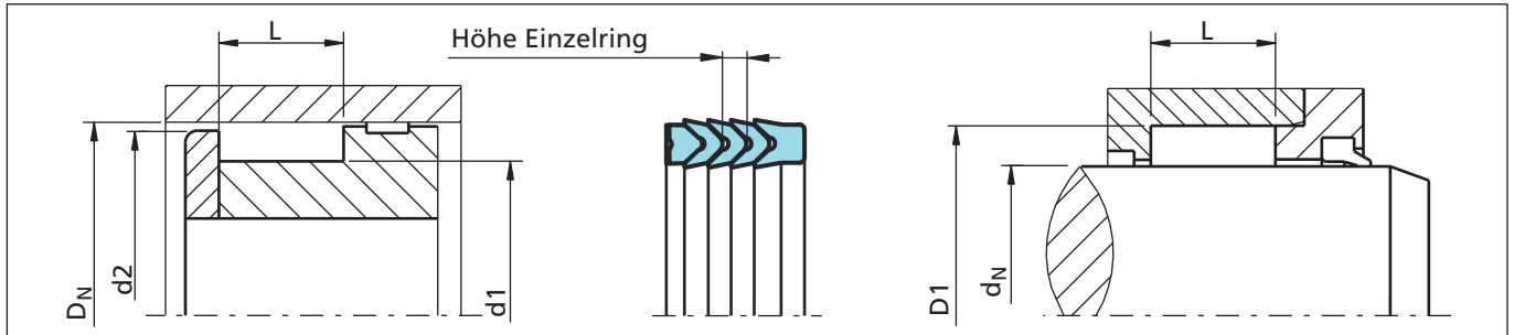
Bild 30 Einbauzeichnung
