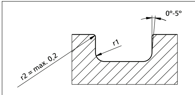
Bild 15 Nutausführung
