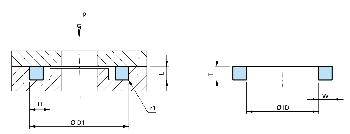
Bild 16 Einbauzeichnung
