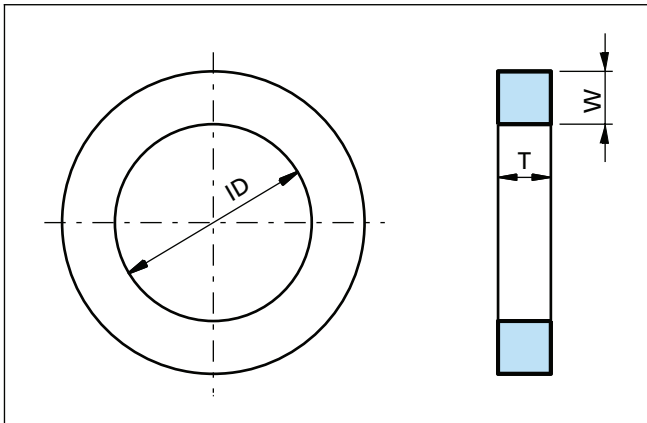
Bild 13 Kantseal Bemaßung
